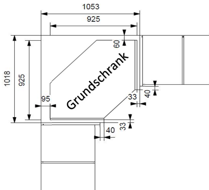
45° Ecke, 1-türig
