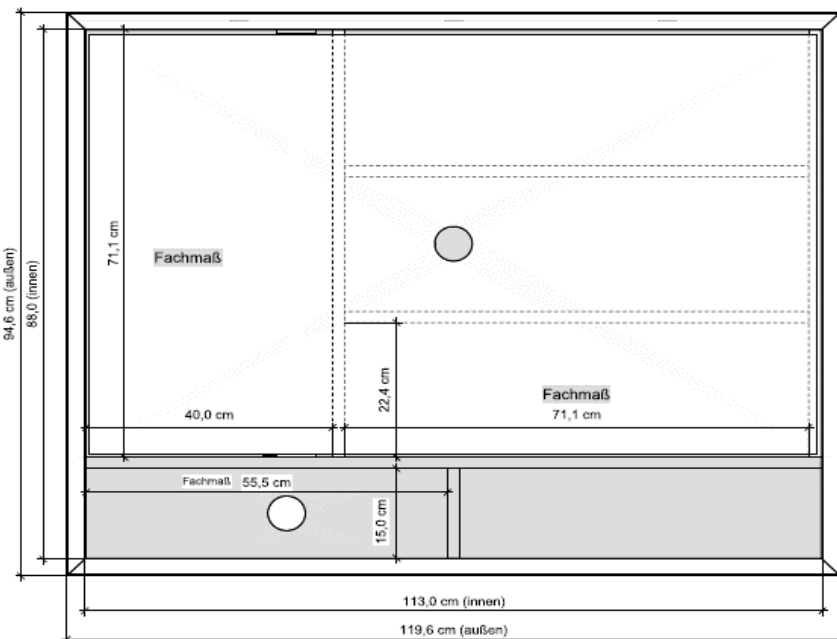
Panel schwenkbar links oder rechts Ansicht geschlossen
